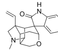
Gelsemine
