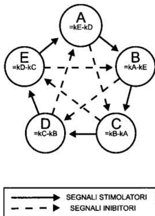
Figura 18. Rappresentazione schematica della rete a cinque nodi variabili di continuo utilizzata per le simulazioni al computer.
