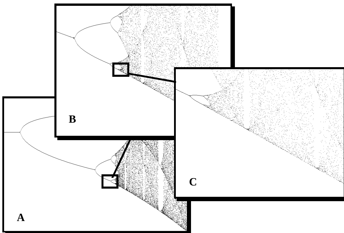
Figura 10. Il diagramma di biforcazione illustrato in figura 9 mostra la classica simmetria dell'invarianza di scala.
