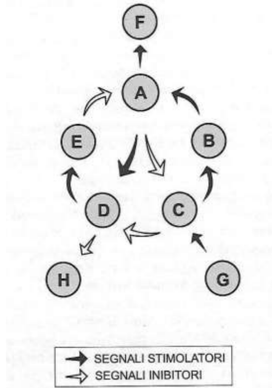
Figura 41. Modello di una tipica rete omeodinamica di cinque nodi tra cui esiste una relazione di controlli attivatori o inibitori.
