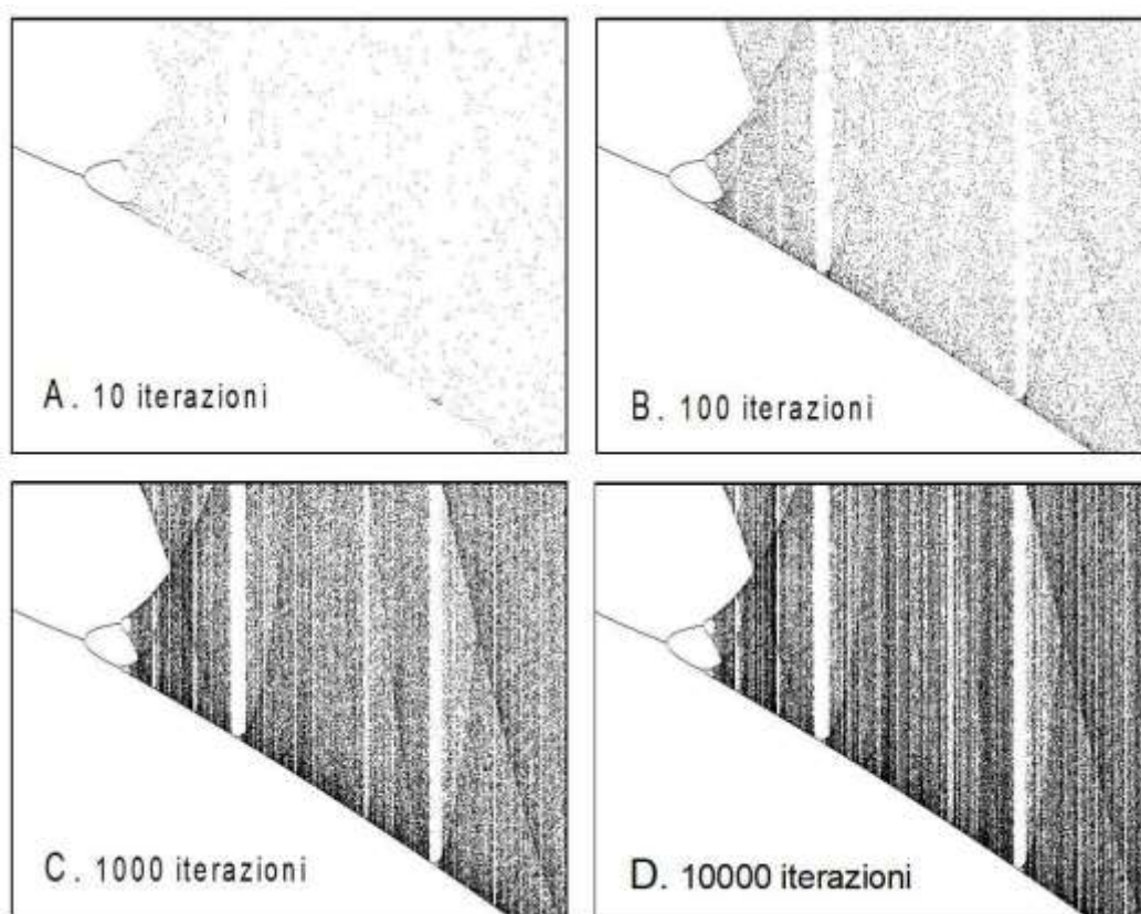
Figura 11. Diagramma di biforcazione della funzione di Verhulst precedentemente descritta, eseguito con diverso numero di iterazioni.
