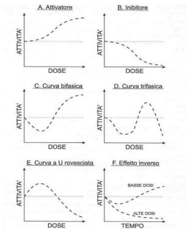
Figura 28. Curve dose-risposta tipiche e atipiche, che mostrano il fenomeno della non-linearità, dell’“ormesi” e dell’effetto “rebound”.
