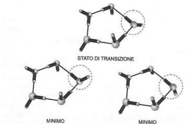
Figura 26. Possibili diverse configurazioni delle molecole d'acqua che formano un pentamero, legate mediante il legame idrogeno.
